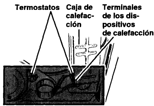
Secadora eléctrica sin el panel posterior
